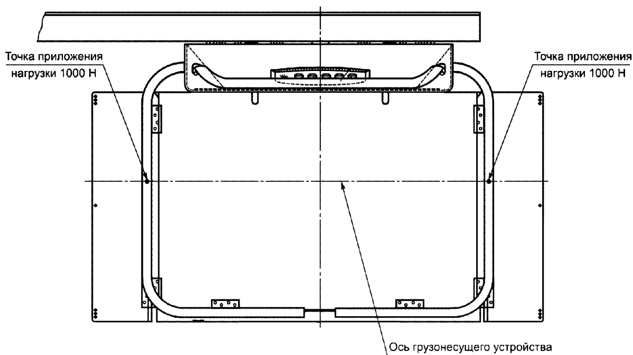
Рисунок Б.4 - Точки приложения нагрузки 1000 Н
