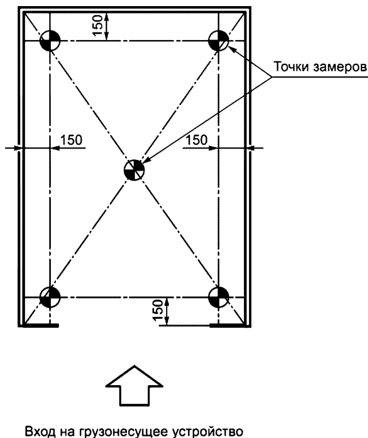
Рисунок Б.2 - Схема расположения контрольных точек
