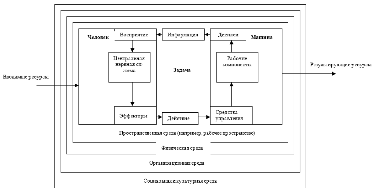
Рисунок 2 – Пример модели системы человек – машина – среда
